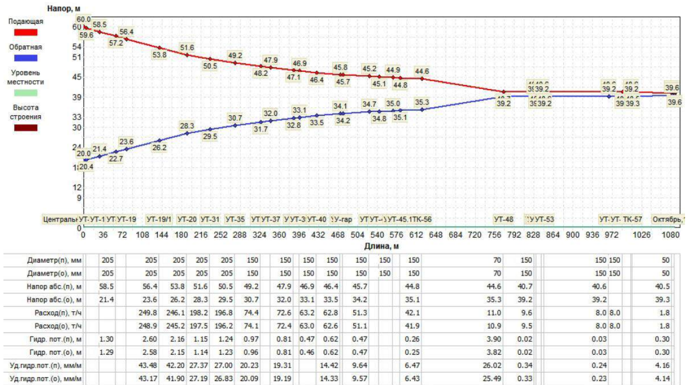
Рис. 9 Пьезометрический график от Центральной котельной до потребителя ул. Октябрьская 1
