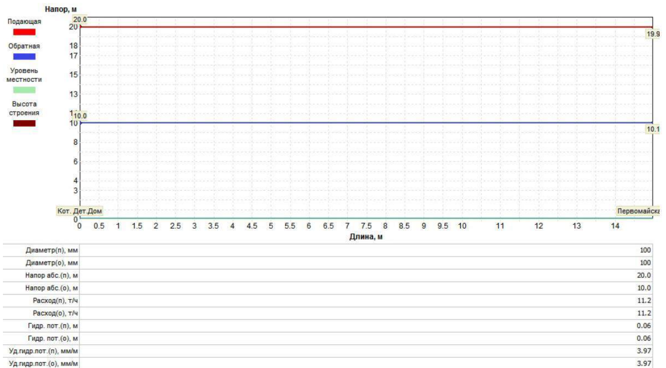
Рис. 12 Пьезометрический график от котельной Детского дома до потребителя Детский дом
