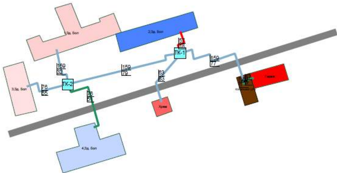
Рис. 16 Гидравлическая схема котельной ЦРБ.
