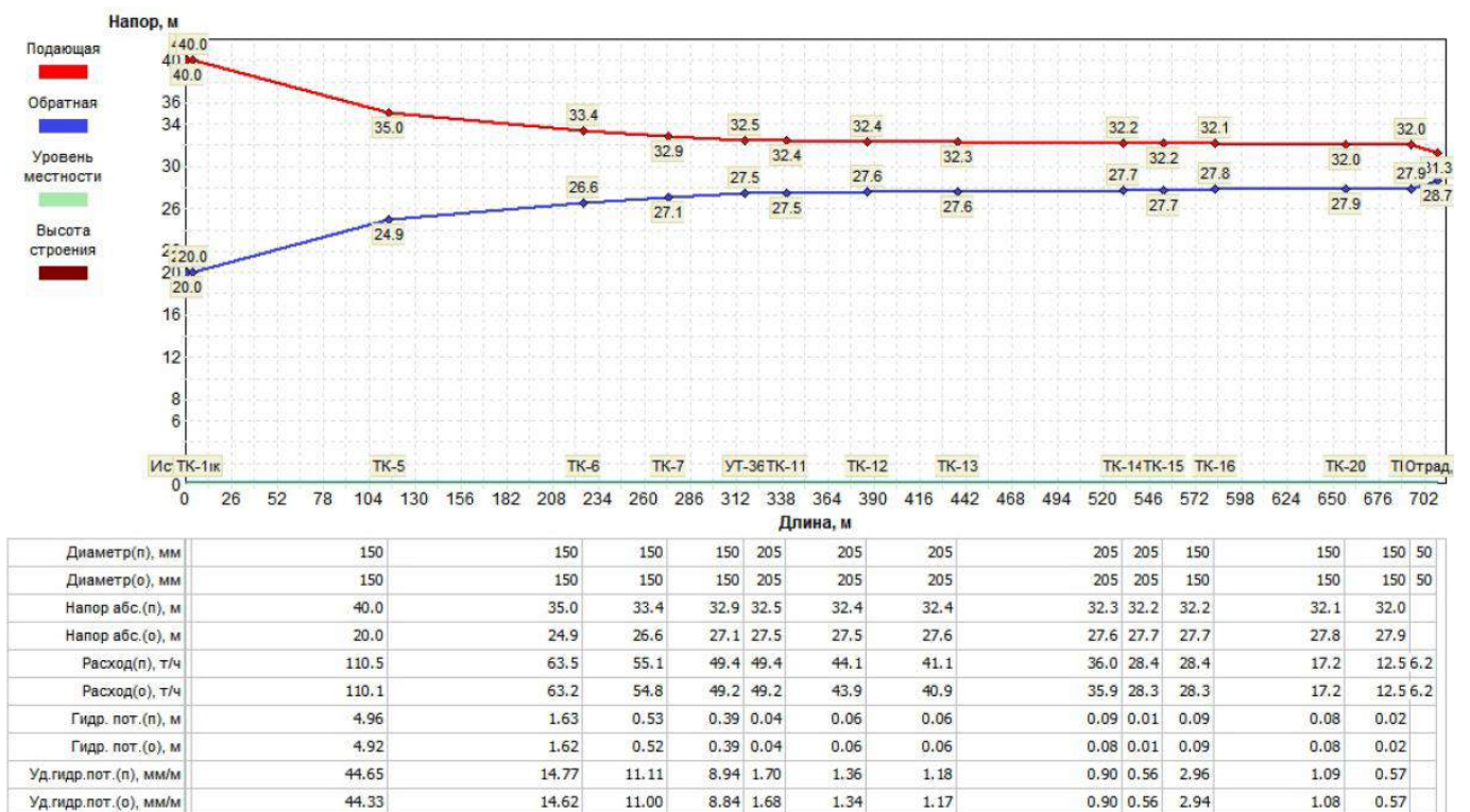
Рис. 11 Пьезометрический график от котельной п. Отрадный до потребителя
