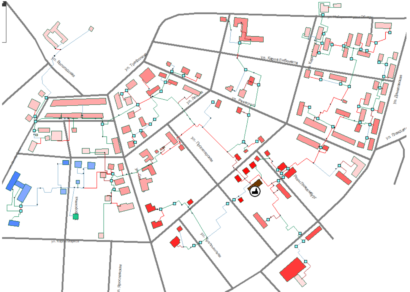
Рис. 36 Гидравлическая схема Центральной котельной.
