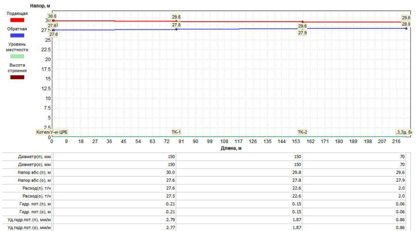
Рис. 17 Пьезометрический график от котельной ЦРБ до потребителя 3,зд Больницы
