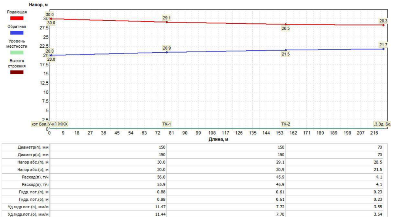
Рис. 10 Пьезометрический график от котельной ЦРБ до потребителя
