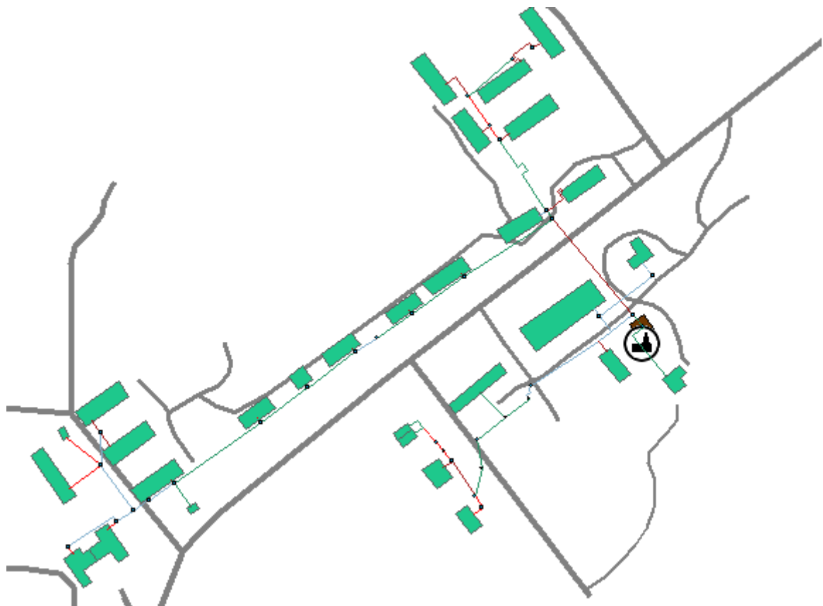
Рис. 24 Схема тепловых сетей с зонами ненормативной надежности от котельной п. Отрадный.
